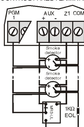
Obr. 9: Čtyř drátové zapojení
