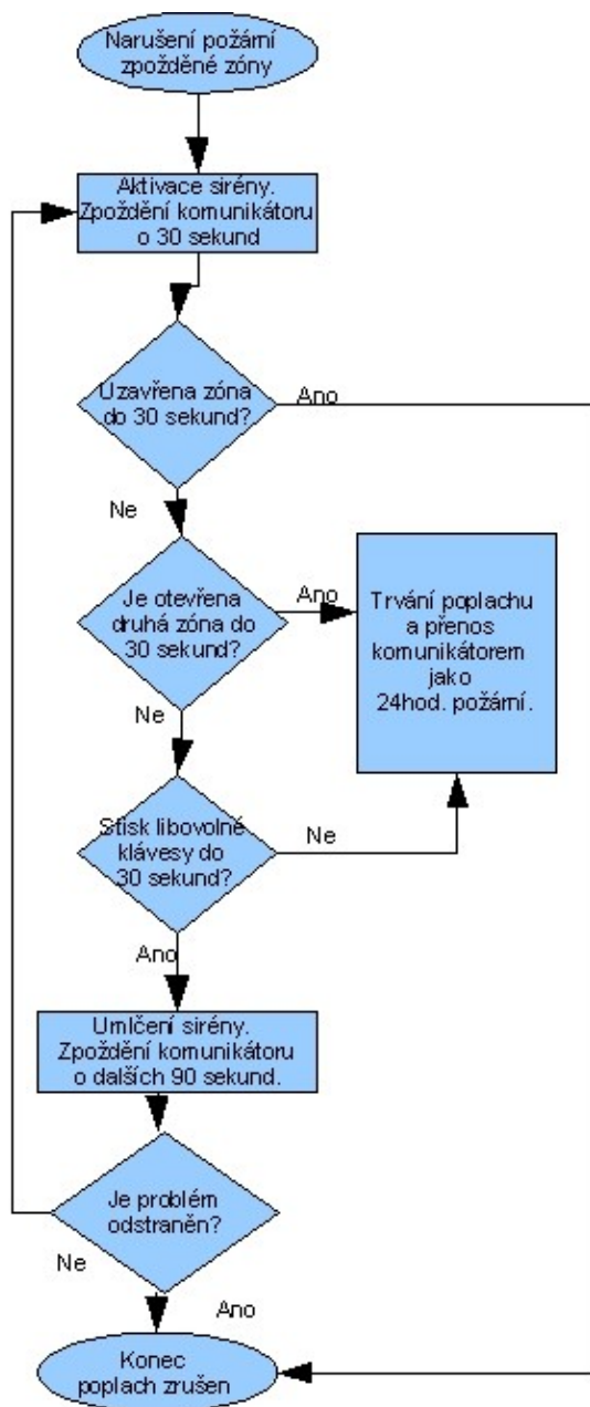
Obr. 14: Zpožděná požární zóna
